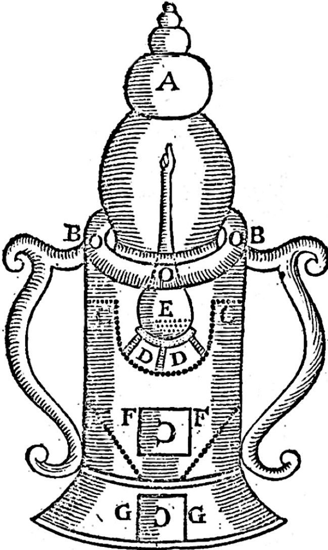
Dieser sub schemate stehende Ofen wird von Kupfer oder Topf gemacht, welcher mit einer Lampe gefeuert werden kann. A ist der Deckel; BB die Register; CC eine kupferne oder blecherne Kapelle; DD ein Dreyfuß, worauf man die Phiole stellet; E die Phiole; FF eine Oefnung, welche unten einen Rost hat, um die Lampe herein zu setzen; GG wieder eine Oefnung unter dem Rost.
